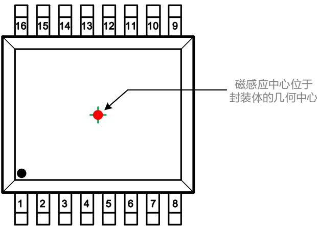
图-1: MT6825 TSSOP-16封装外观图
