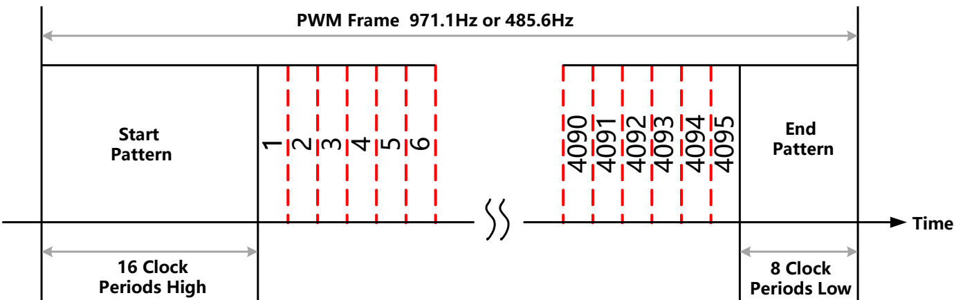
图-13: PWM输出
