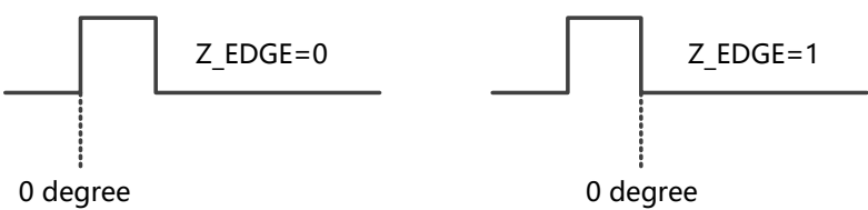
图-13: Z 脉冲的沿和零位的关系
